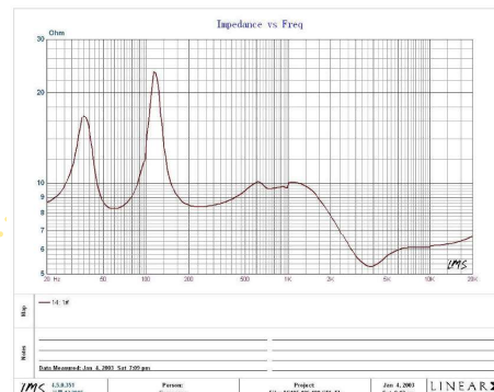
Impedance/Phase
